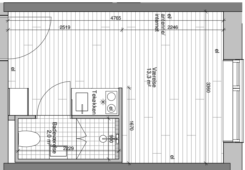
Boligtype A2 - 1 : 50
