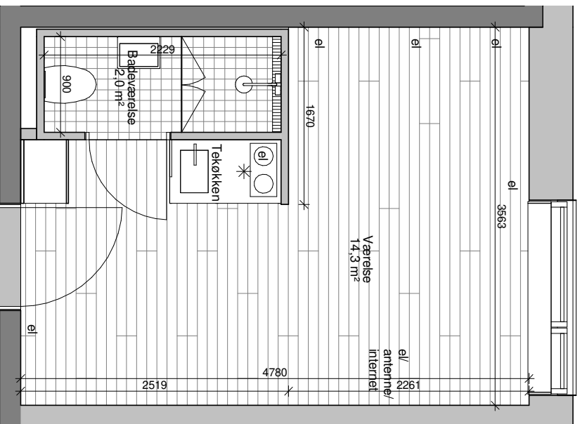
Boligtype A3 - 1 : 50
