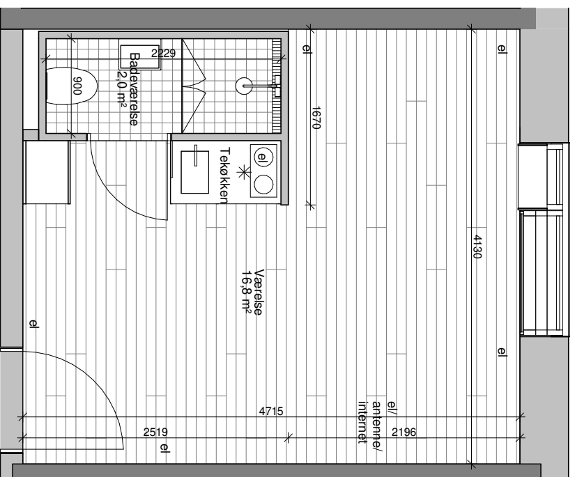
Boligtype A5 - 1 : 50
