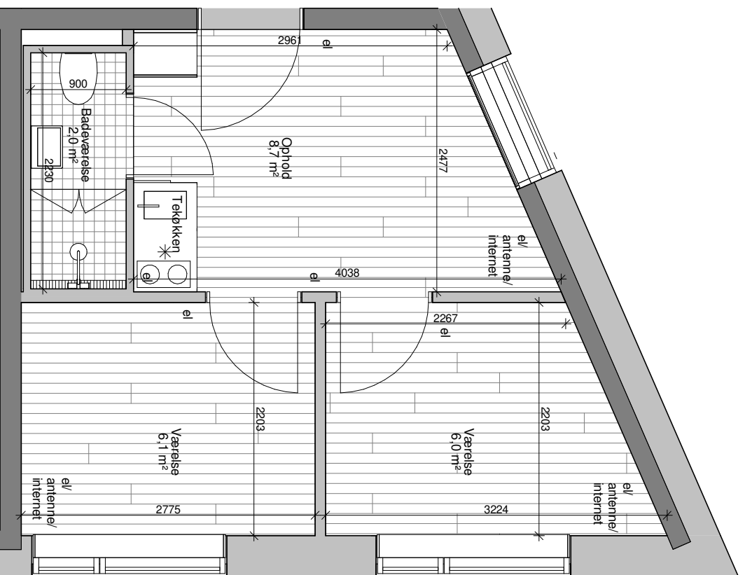
Boligtype B2 - 1 : 50
