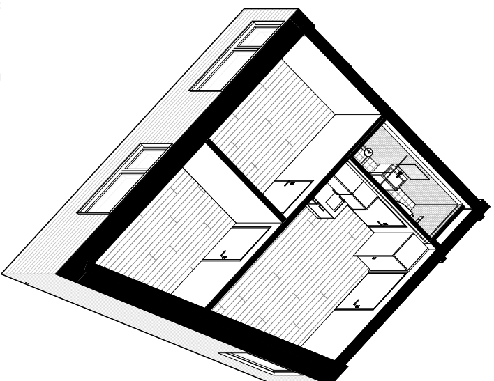
Boligtype B2 - 1 : 50
